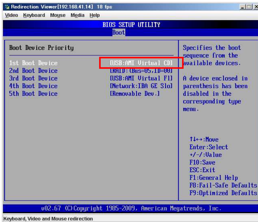
図 6 起動順序の変更(2)
