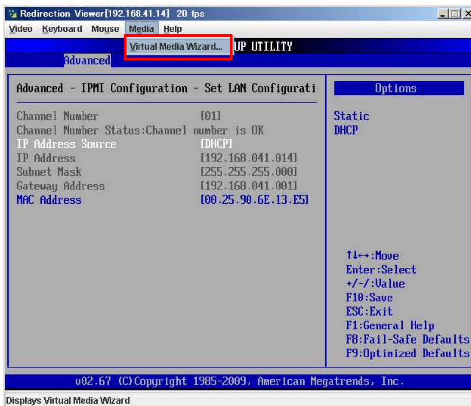
図 2 Virtual Media Wizard の起動
