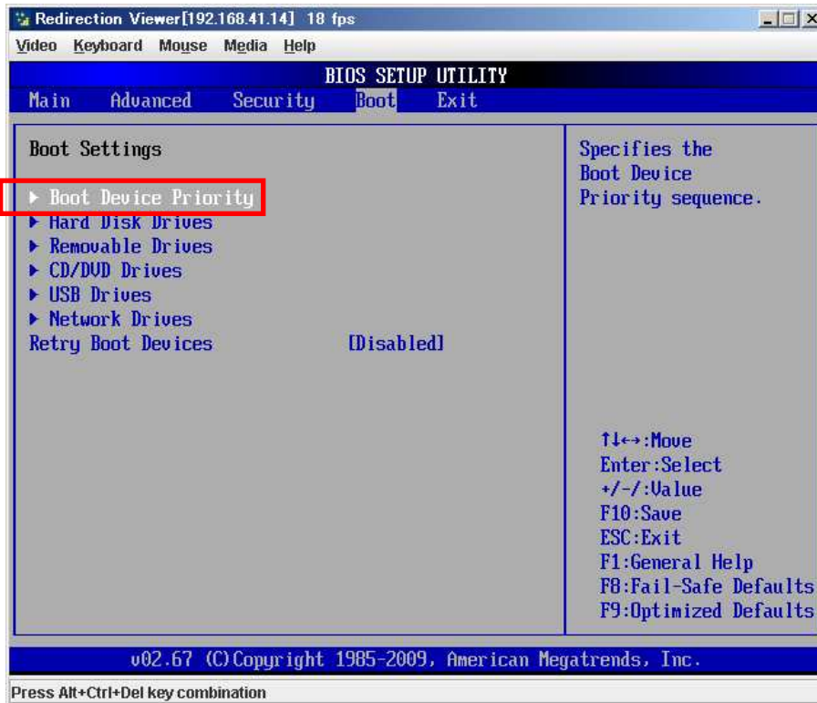
図 5 起動順序の変更(1)
