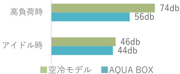
同型の空冷モデルと比較し高い静音性
